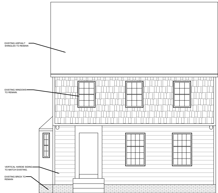
1 EAST ELEVATION A-1 SCALE: 1/8" = 1'-0"
