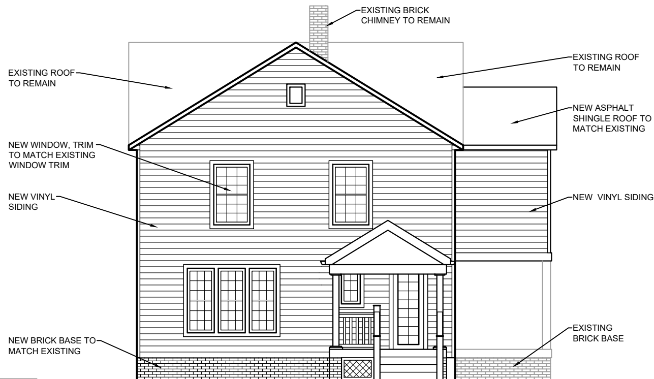
3 2 SOUTH ELEVATION SCALE: 1/8" = 1'-0"
