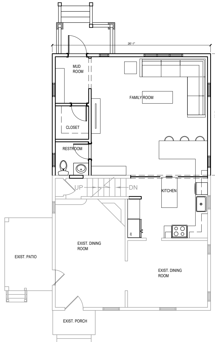
2 A-1 FIRST FLOOR PLAN SCALE: 1/8" = 1'-0"
