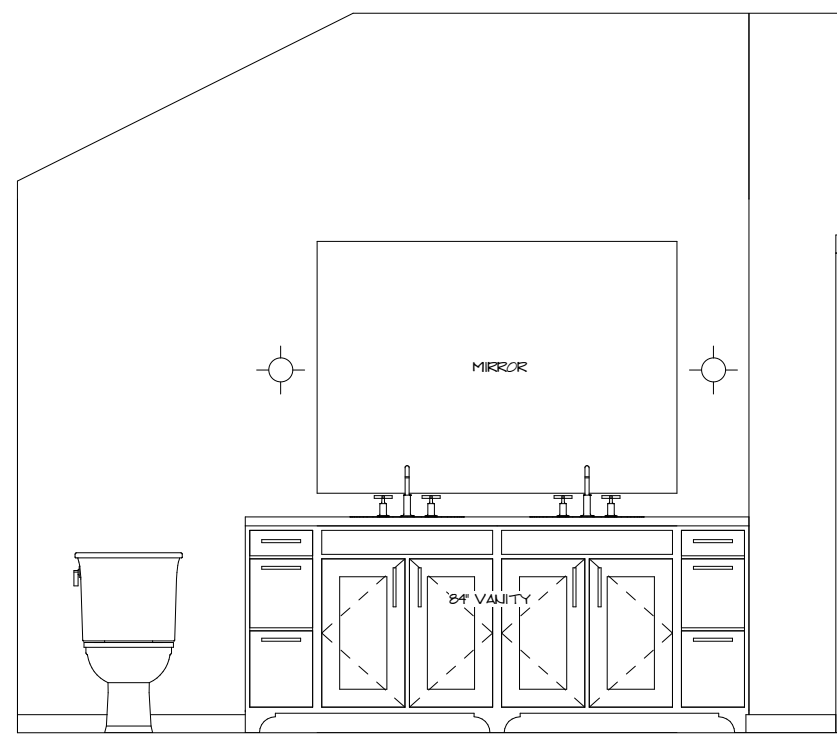
ELE. 3-C 3/8" = 1'-0"
