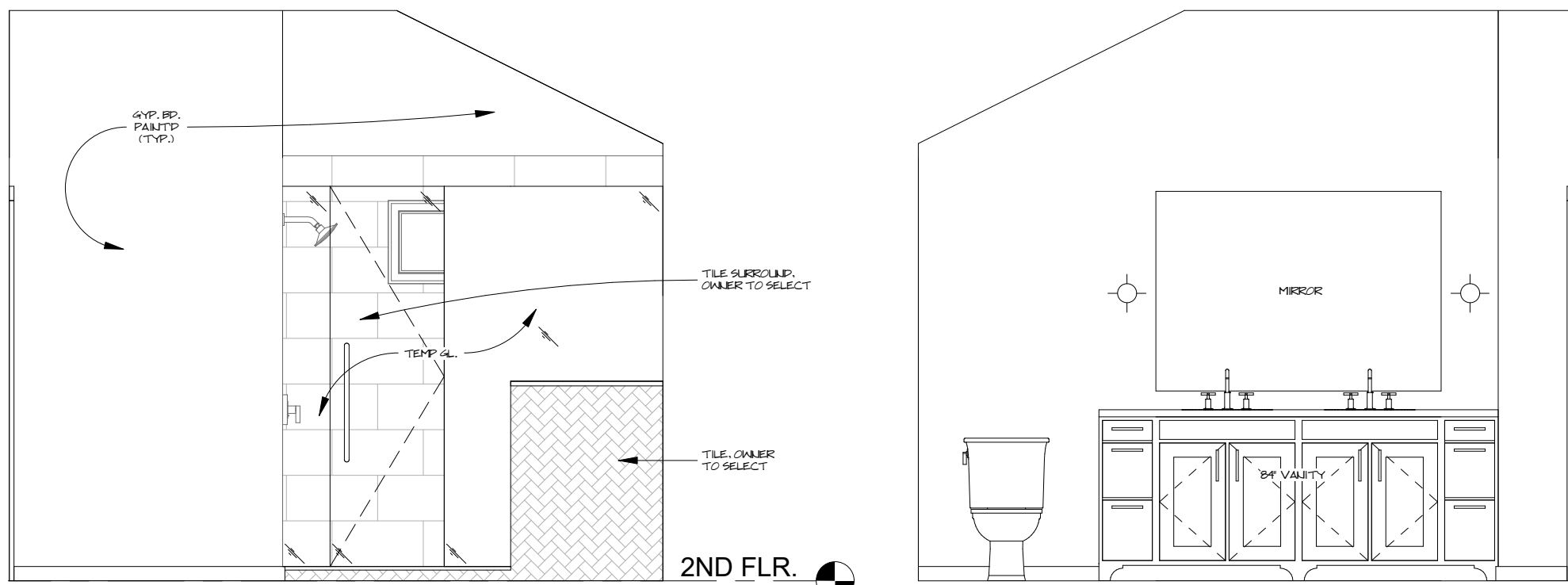
ELE. 3-A 3/8" = 1'-0"
