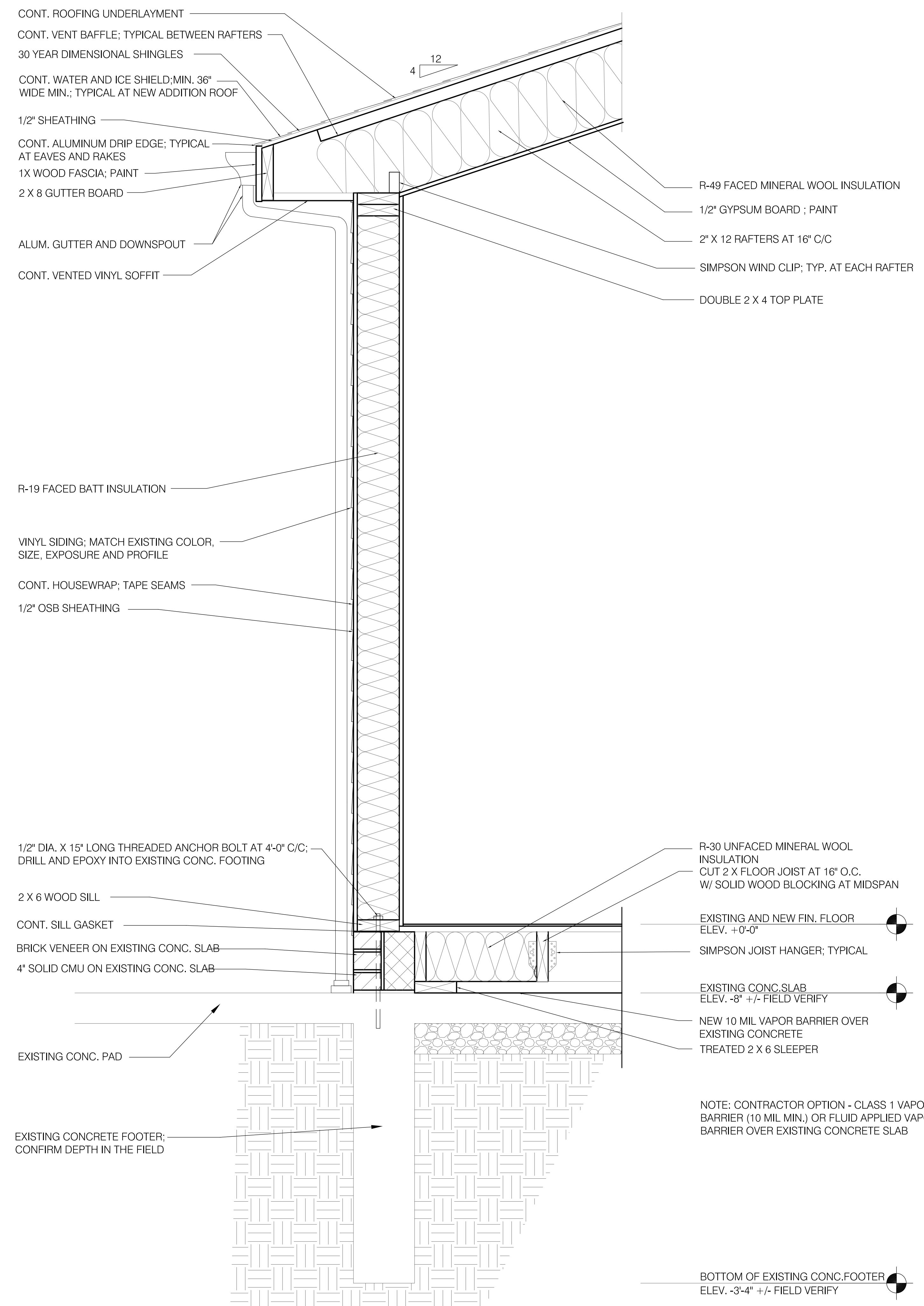
2 WALL SECTION SCALE: 1 1/2"=1'-0"
